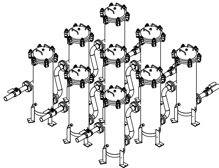
ИЗОМЕТРИЧЕСКИЙ ВИД
